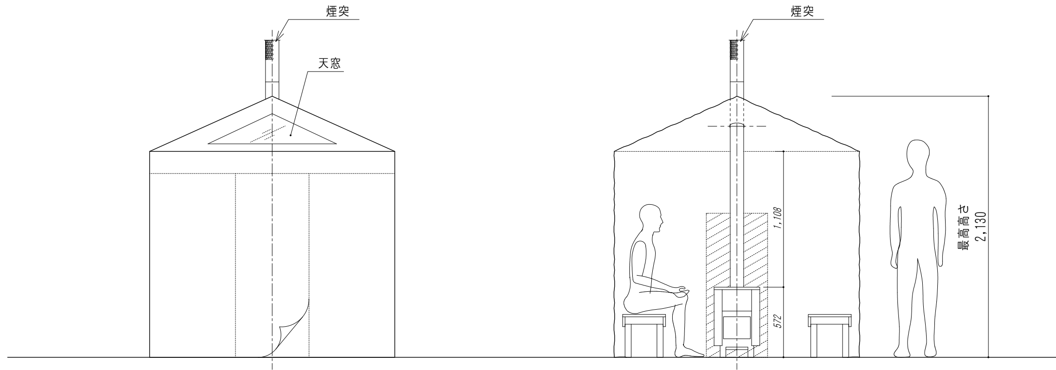
正面図
