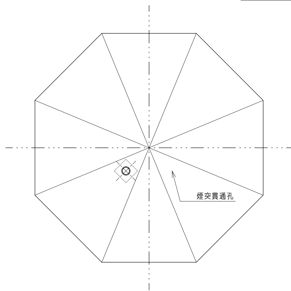
屋根伏図
